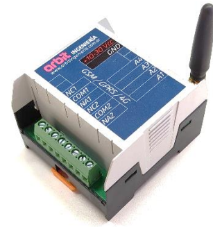
Figura 1. Unidad GSM/GPRS/4G
