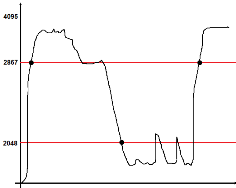
Figura 3. Ejemplo de alarma digital para la entrada 1: 0000,ENT,1,2,1,0,1,0,
